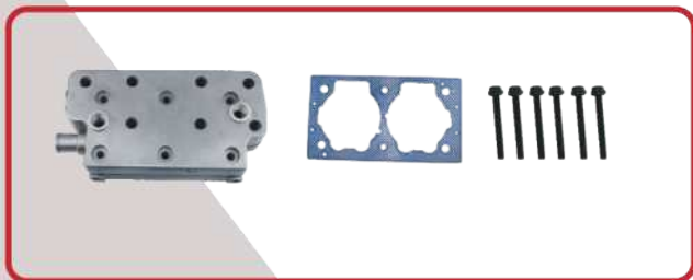
WABCO 911 515 003 0
