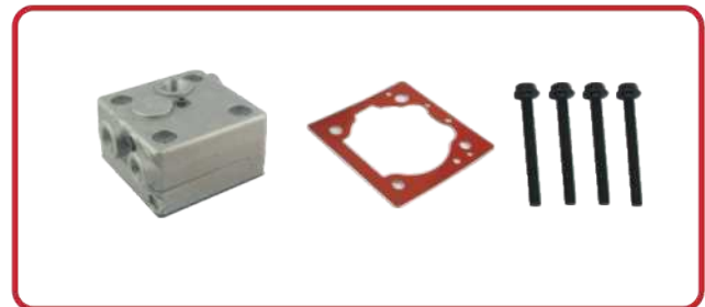
WABCO 911 155 512 0 911 155 511 0
